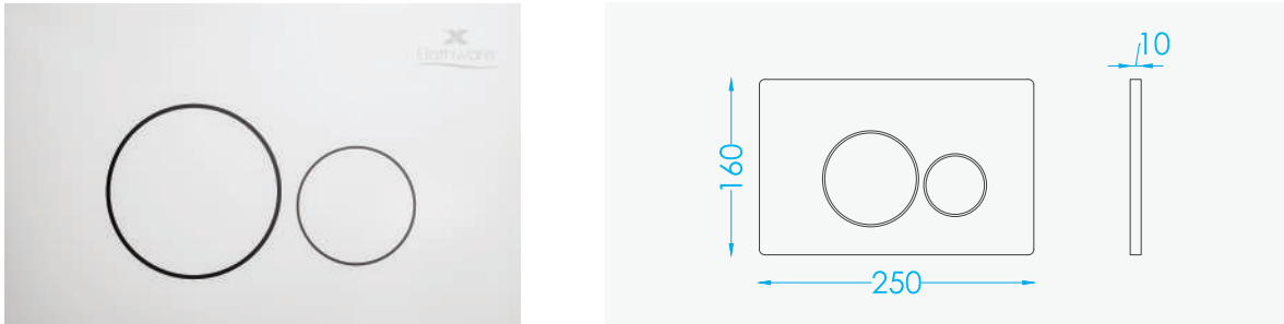
PUSH PLATE (W250 L/H160)
